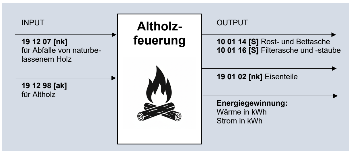
Abbildung 1: Vereinfachtes Schema der häufigsten Stoffflüsse bei Altholzfeuerungen, Input in Schnitzelform
